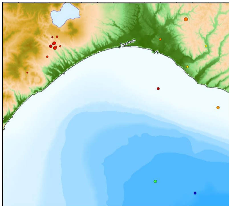
2016年6月の自然地震震源分布
