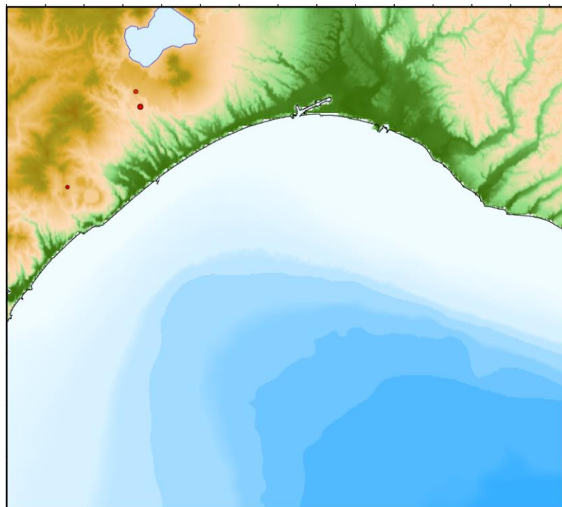
2016年9月の自然地震震源分布
