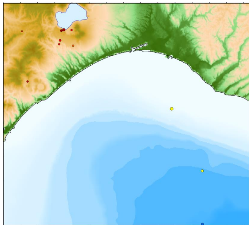
2016年10月の自然地震震源分布
