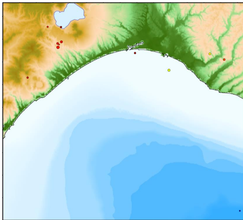
2017年1月の自然地震震源分布
