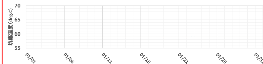
滝ノ上層観測井OB-3 平均値：58.9°C(深度1743m)
