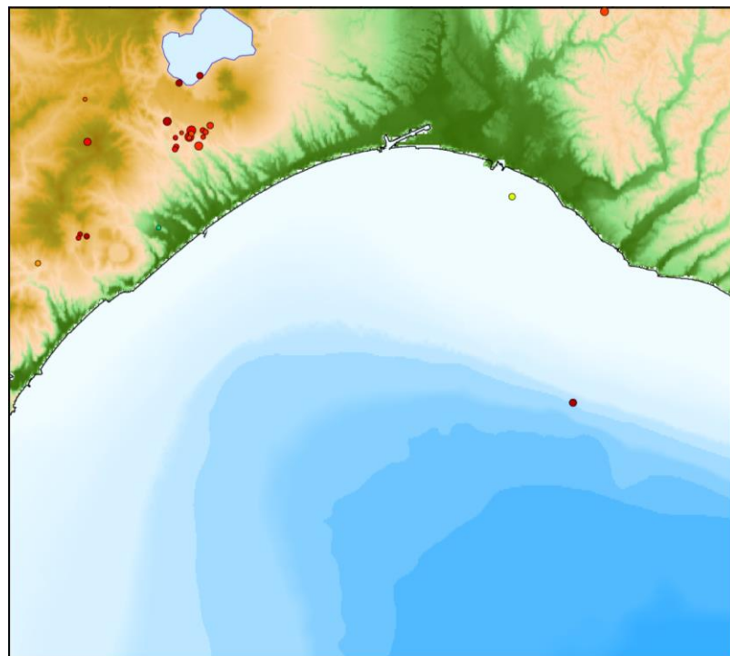
2017年3月の自然地震震源分布
