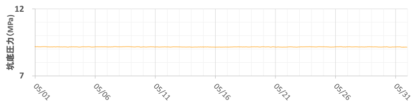
萌別層観測井OB-2 平均値：9.16MPa(深度893m)
