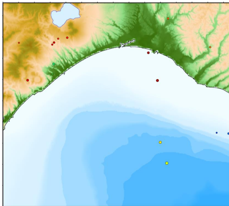
2017年5月の自然地震震源分布
