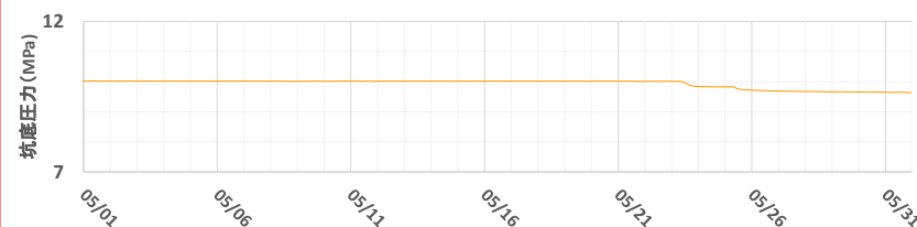
萌別層圧入井 平均値：9.93 MPa(深度930m)
