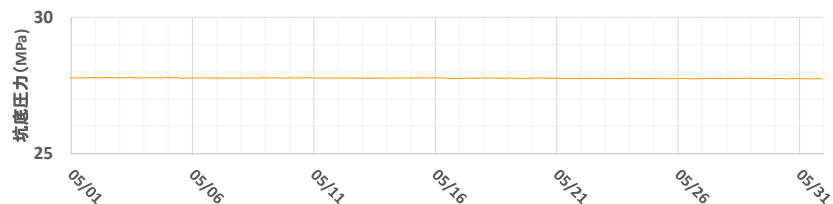
滝ノ上層観測井OB-1 平均値：27.79MPa(深度2003m)
