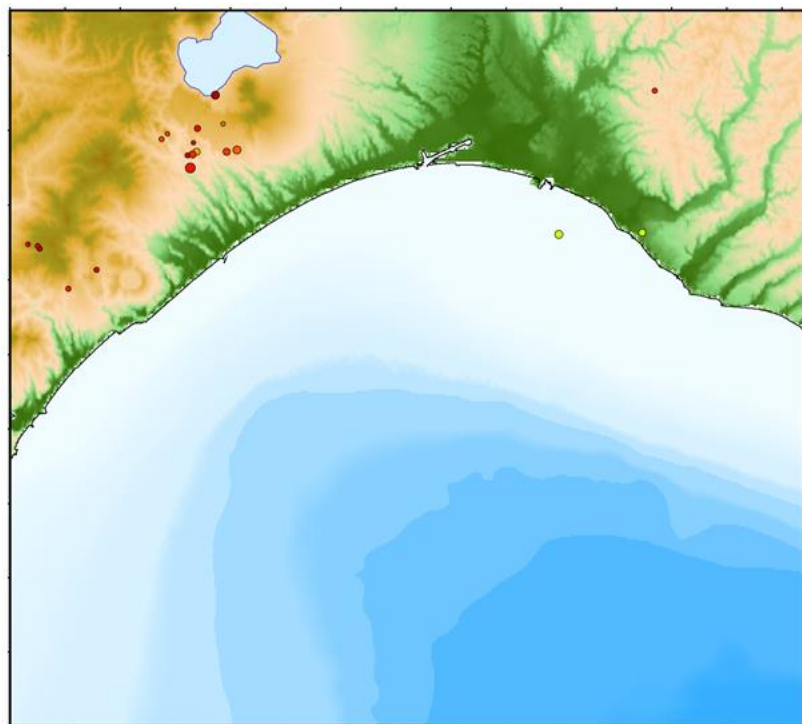
2017年6月の自然地震震源分布
