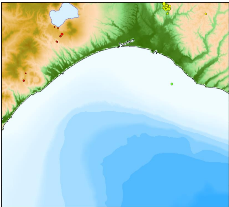
2017年8月の自然地震震源分布
