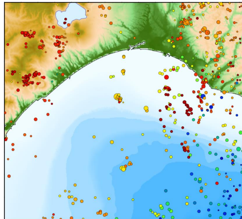
2001年～2010年に発生した自然地震震源分布
