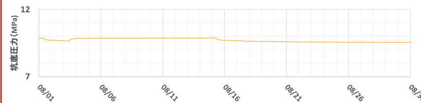
萌別層圧入井 平均値：9.70 MPa(深度930m)
