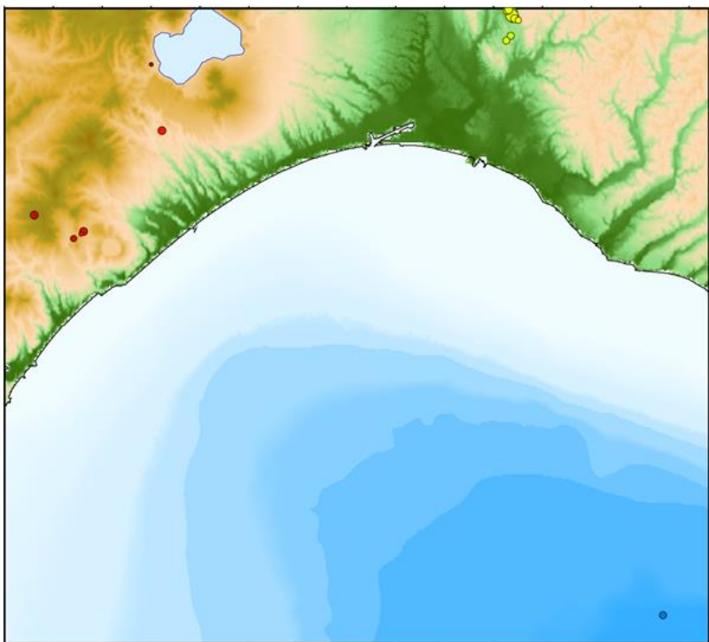
2017年9月の自然地震震源分布
