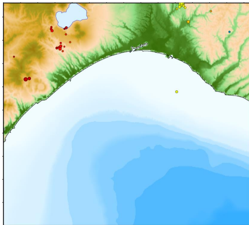
2017年10月の自然地震震源分布
