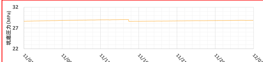
滝ノ上層観測井OB-3 平均値：28.77MPa(深度1743m)
