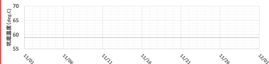
滝ノ上層観測井OB-3 平均値：58.9°C(深度1743m)
