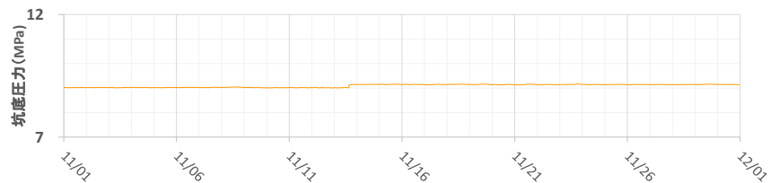
萌別層観測井OB-2 平均値：9.09MPa(深度893m)
