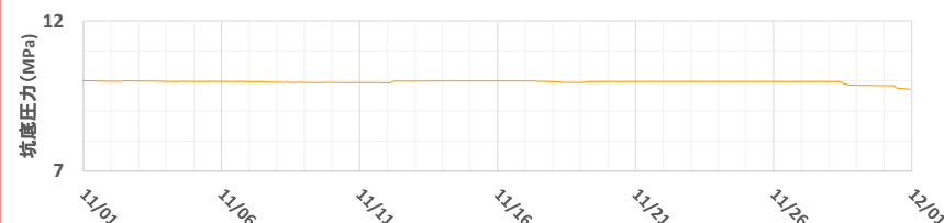
萌別層圧入井 平均値：9.97 MPa(深度930m)
