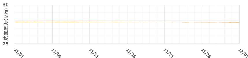
滝ノ上層観測井OB-1 平均値：27.78MPa(深度2003m)
