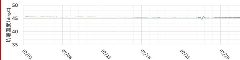
萌別層圧入井 平均値：45.5°C(深度930m)
