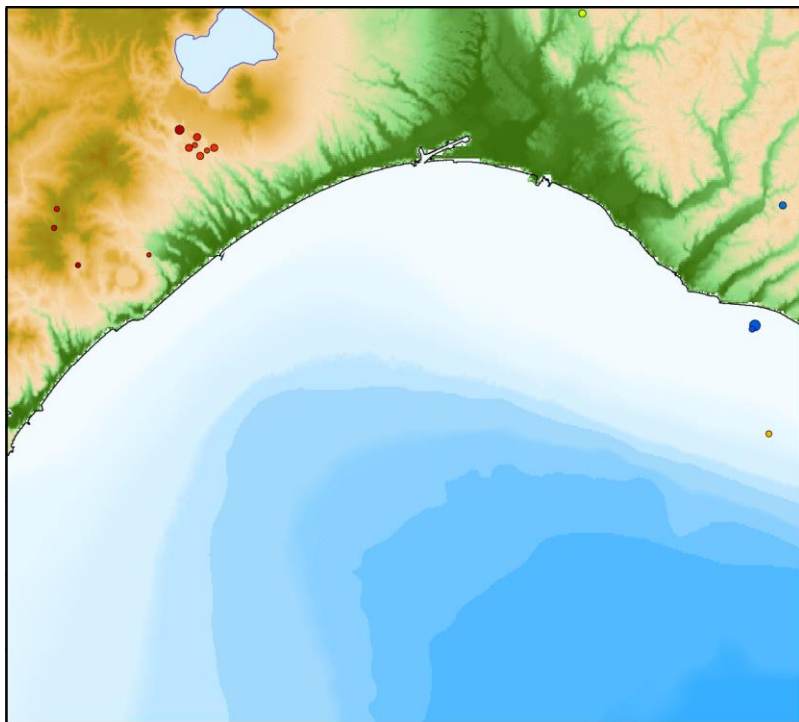
2018年5月の自然地震震源分布
