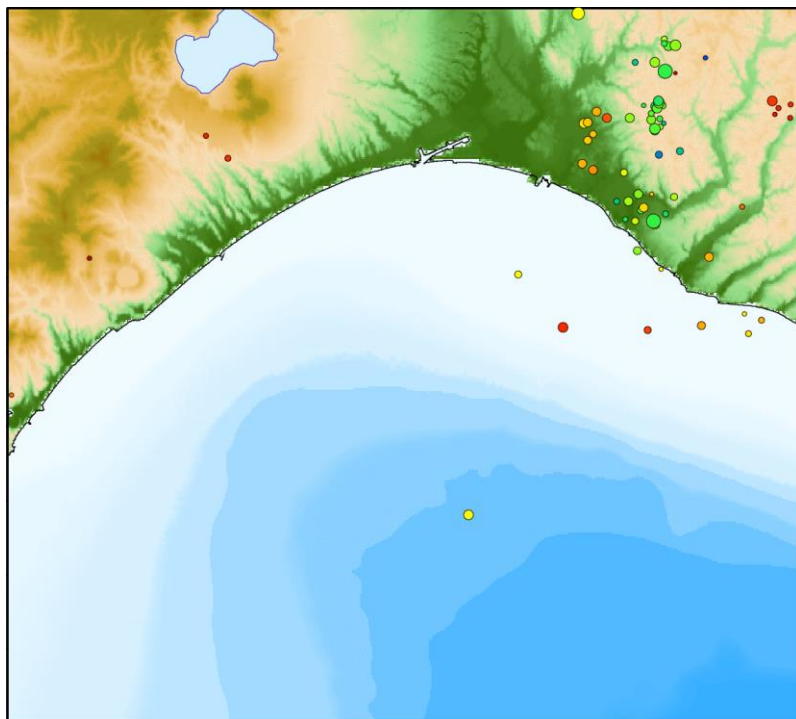
2019年5月の自然地震震源分布
