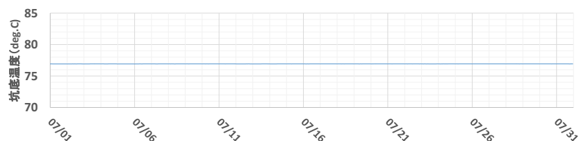
滝ノ上層観測井OB-1 平均値：76.9°C(深度2003m)
