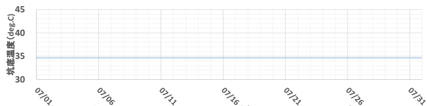
萌別層観測井OB-2 平均値：34.6°C(深度893m)
