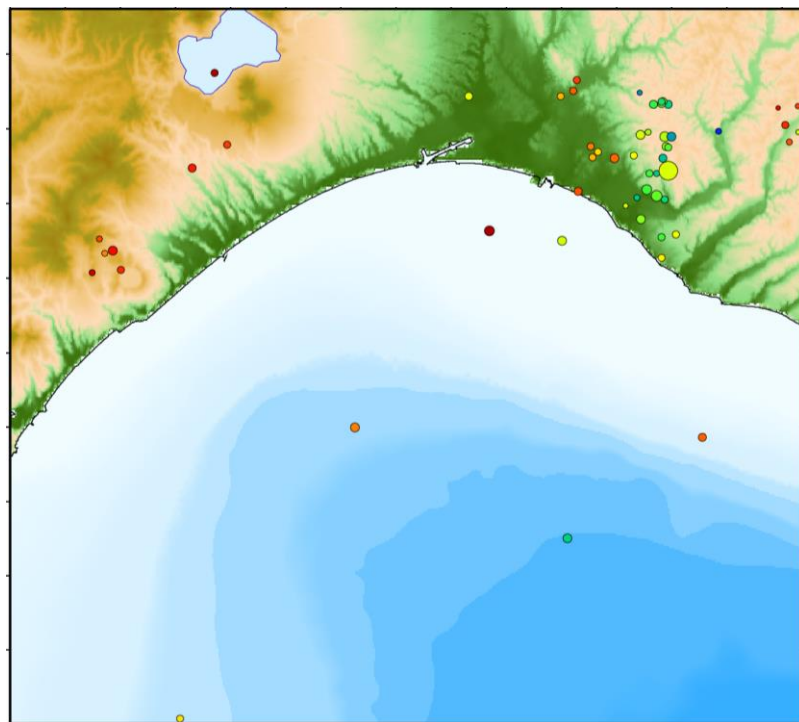
2019年7月の自然地震震源分布
