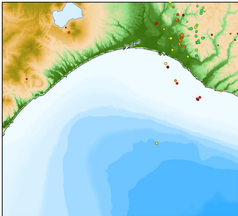
2019年9月の自然地震震源分布
