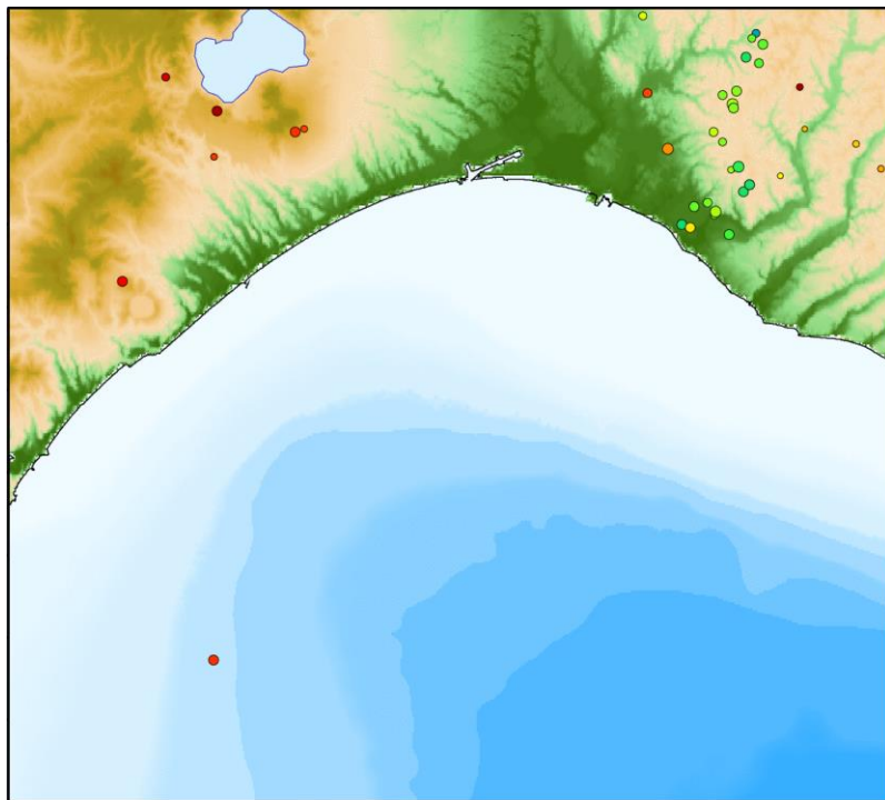
2019年10月の自然地震震源分布
