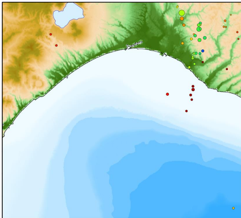
2019年12月の自然地震震源分布
