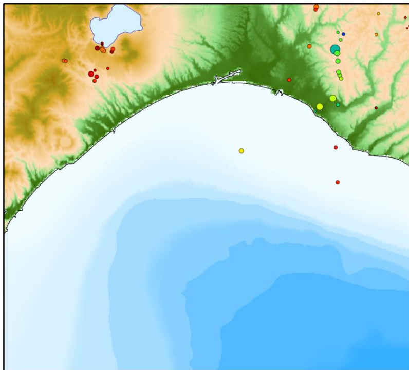
2020年2月の自然地震震源分布
