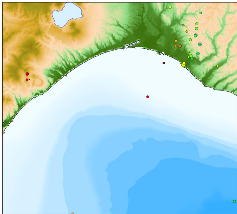
2020年4月の自然地震震源分布
