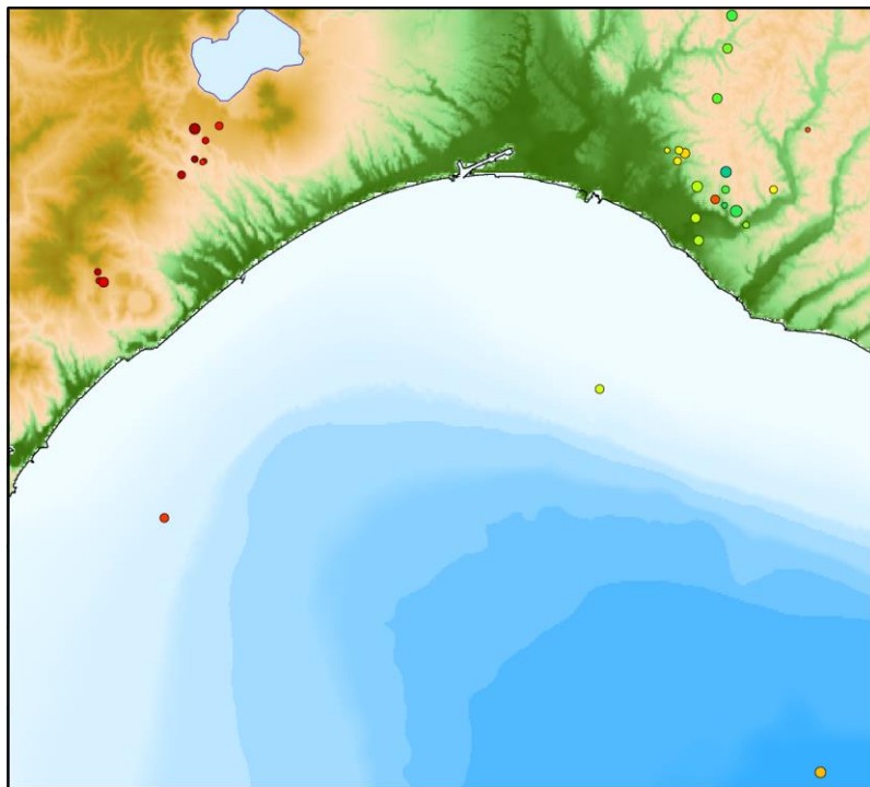
2020年5月の自然地震震源分布
