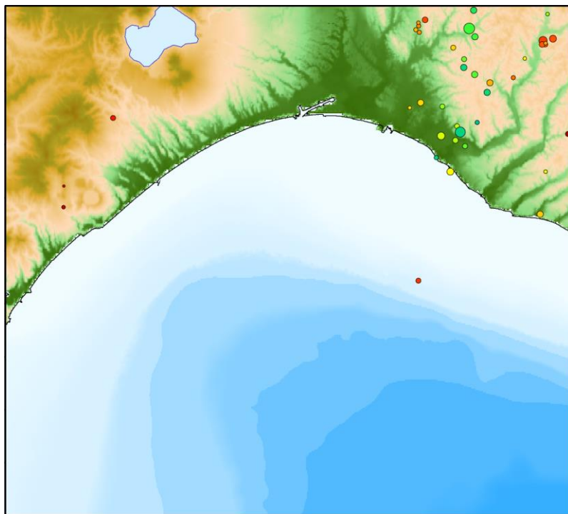
2020年7月の自然地震震源分布
