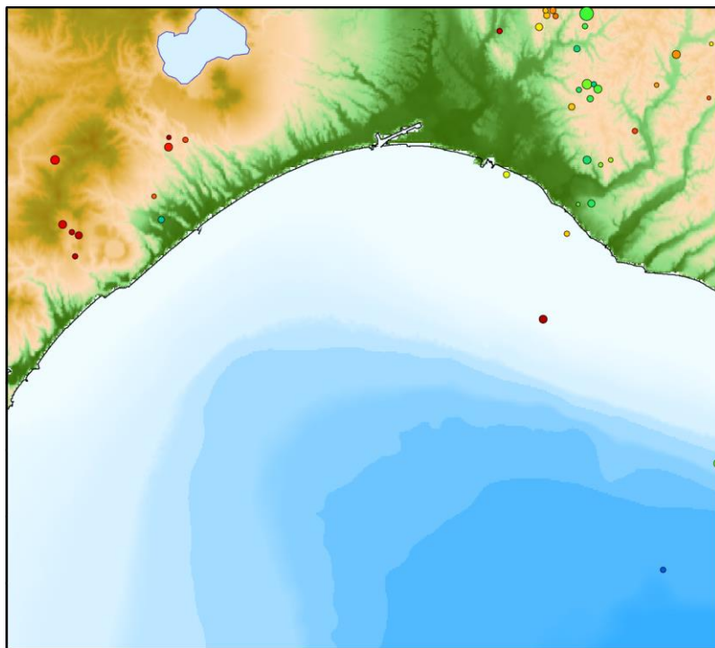
2020年8月の自然地震震源分布
