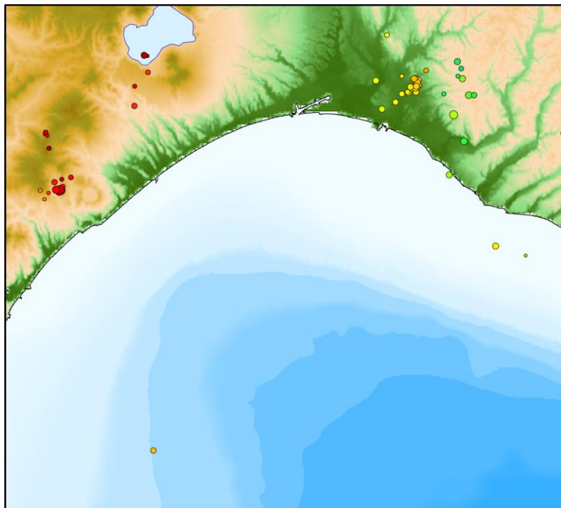
2020年9月の自然地震震源分布
