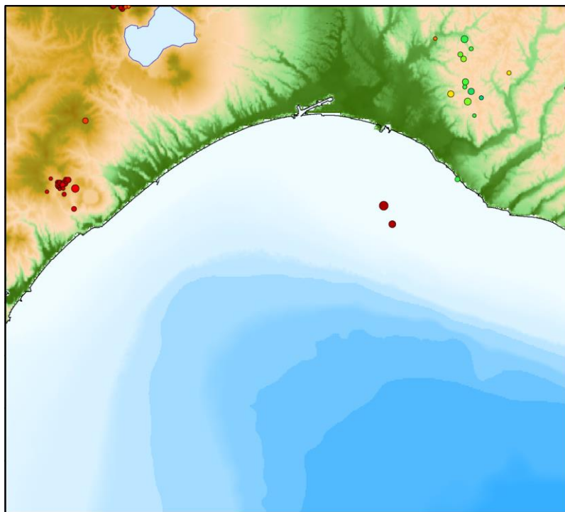
2020年11月の自然地震震源分布
