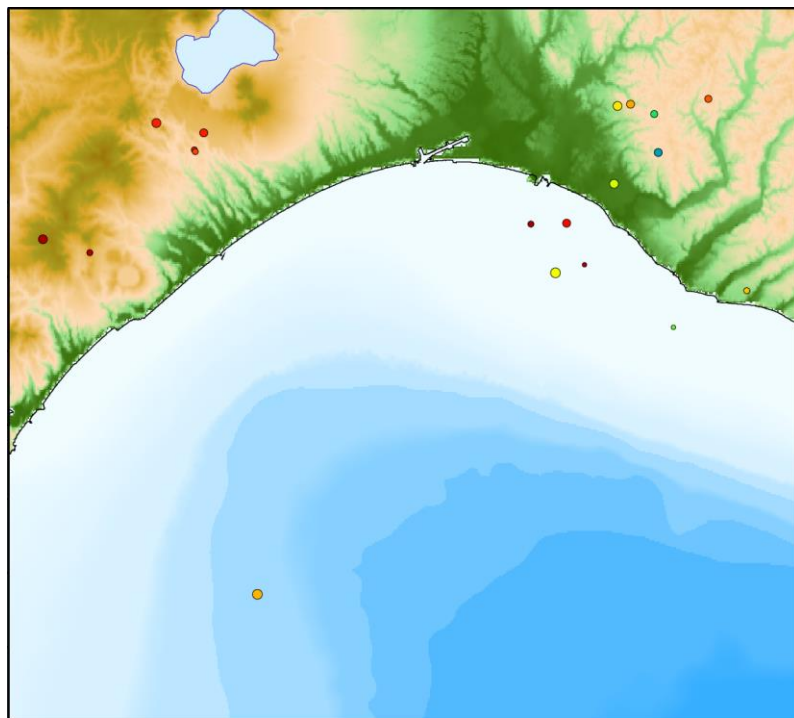
2022年3月の自然地震震源分布
