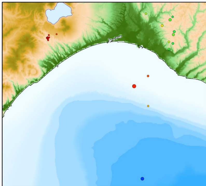
2022年4月の自然地震震源分布
