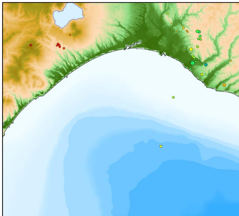
2022年7月の自然地震震源分布
