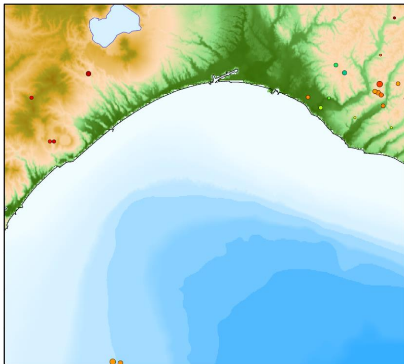
2022年12月の自然地震震源分布
