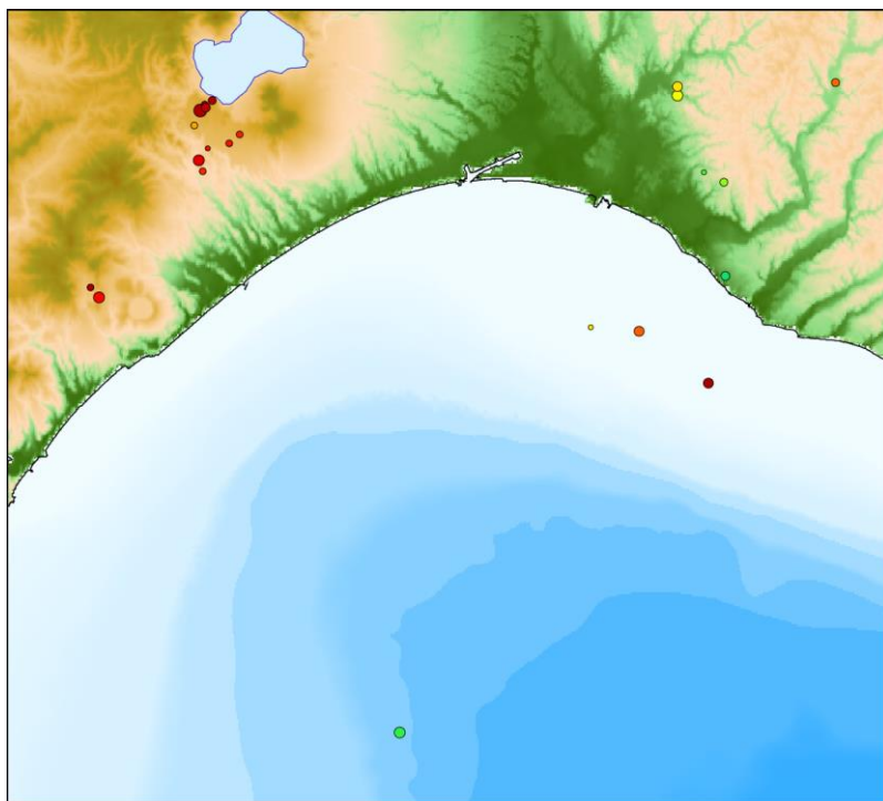
2023年4月の自然地震震源分布
