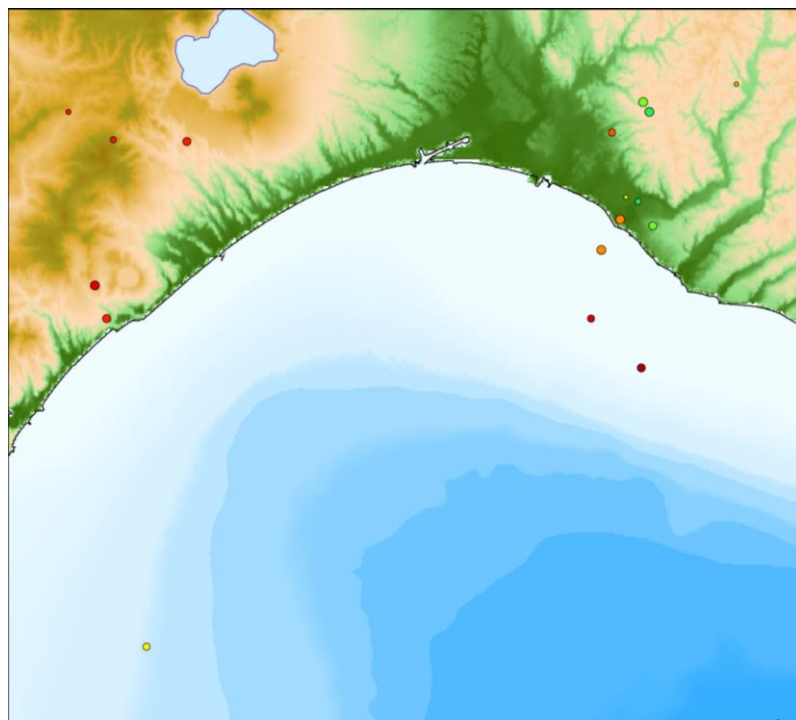
2023年5月の自然地震震源分布
