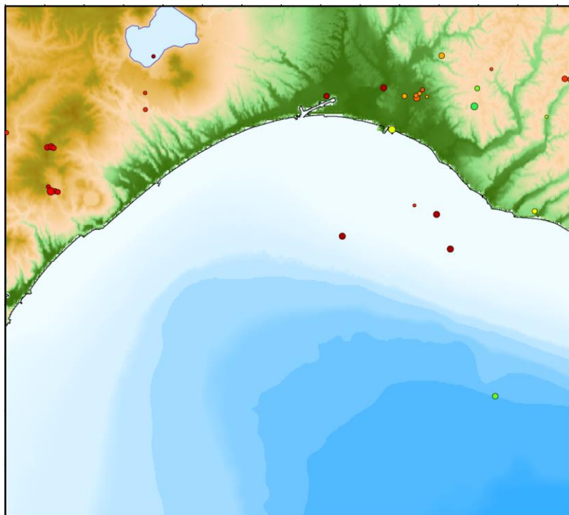
2023年10月の自然地震震源分布
