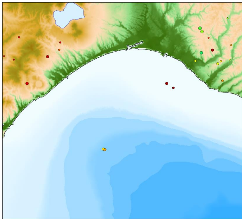
2024年4月の自然地震震源分布
