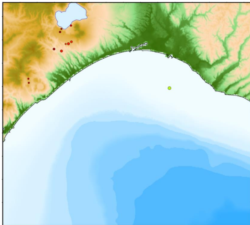
2016年5月の自然地震震源分布
