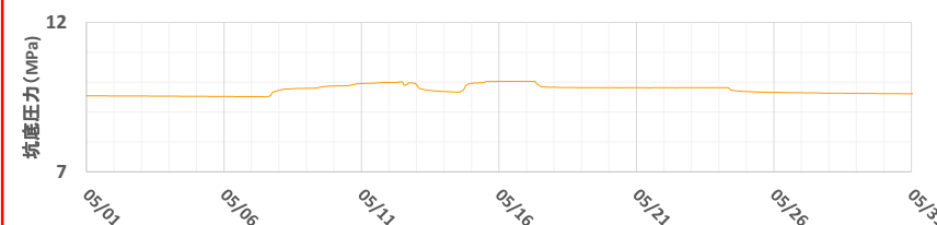
萌別層圧入井 平均値：9.73 MPa(深度930m)
