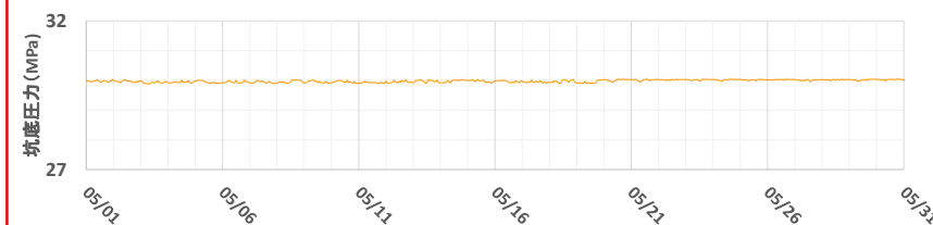
滝ノ上層観測井OB-3 平均値：29.98MPa(深度1773m)
