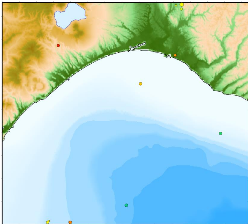
2018年4月の自然地震震源分布
