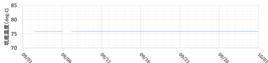
滝ノ上層観測井OB-1 平均値：75.8°C(深度2003m)
