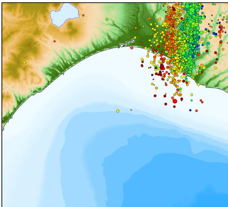
2018年9月の自然地震震源分布
