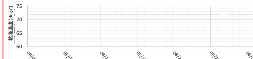
滝ノ上層観測井OB-3 平均値：71.7°C(深度2152.6m)
