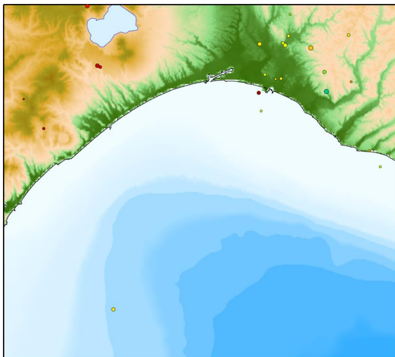
2024年8月の自然地震震源分布
