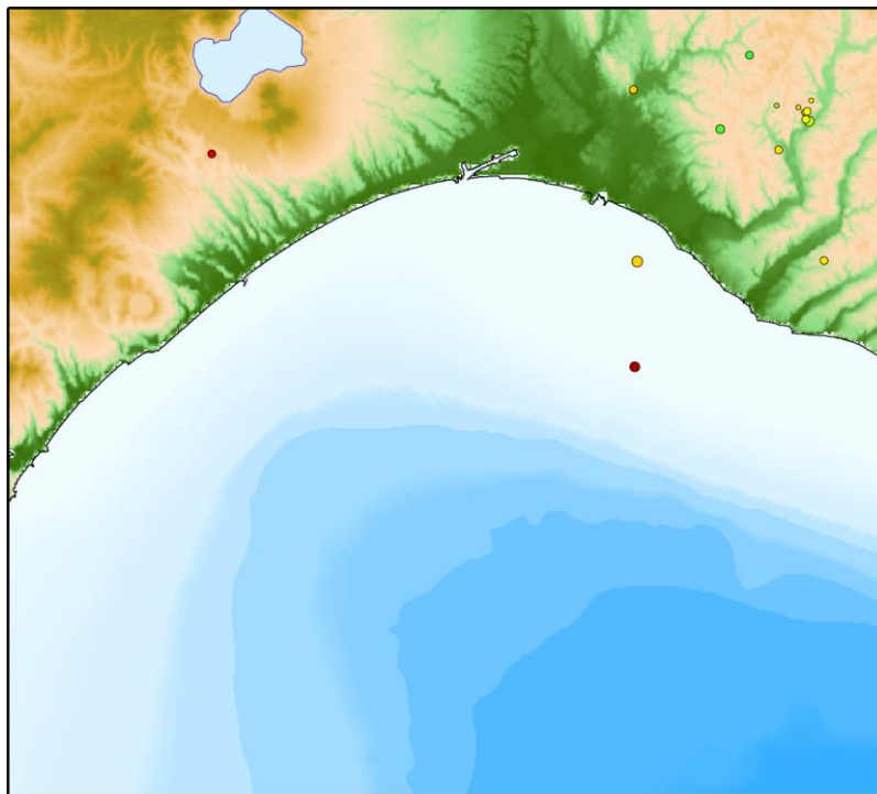
2026年2月の自然地震震源分布
