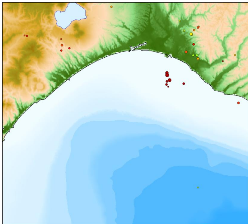
2026年7月の自然地震震源分布
